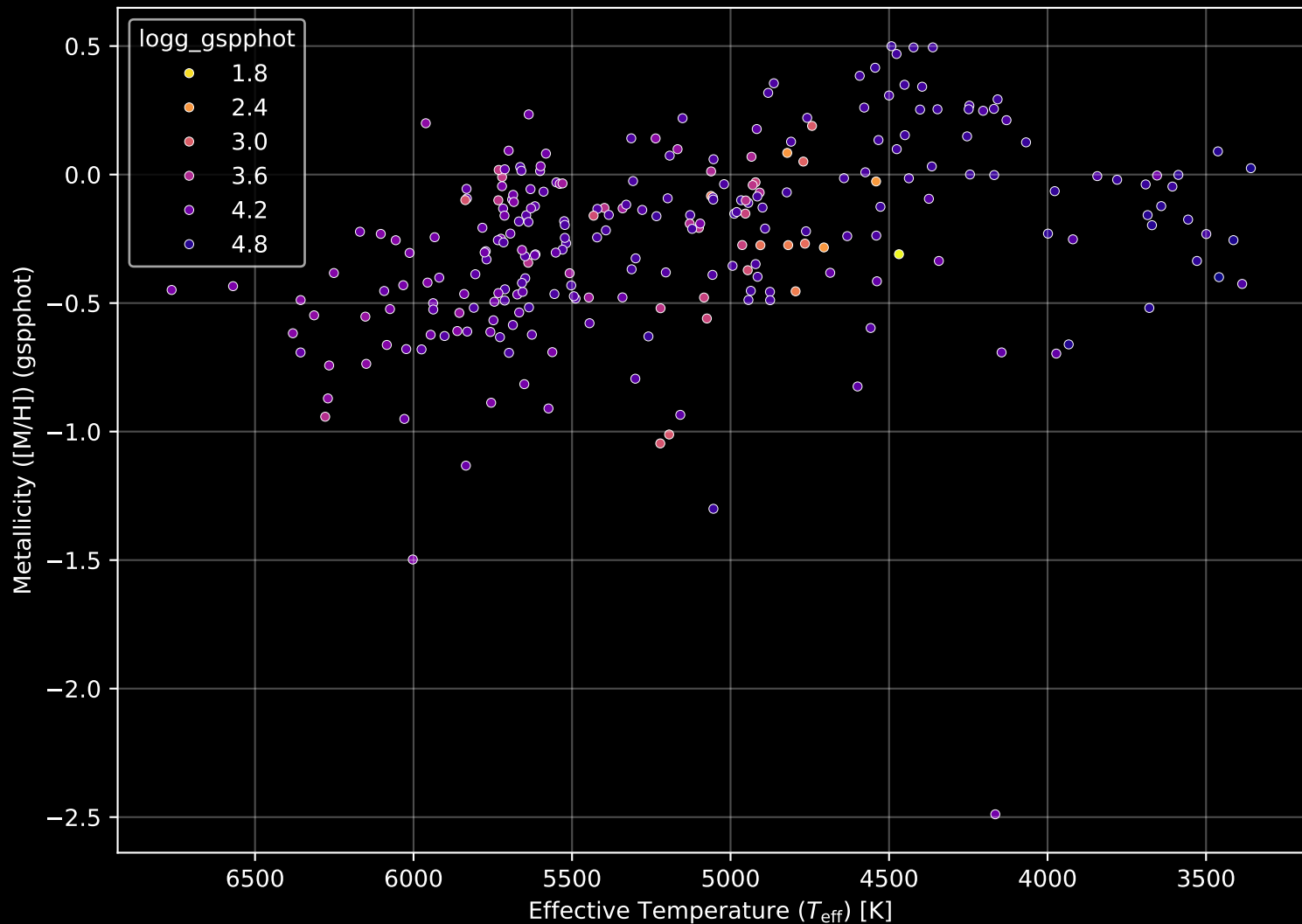
APOGEE DR17 Field: [120-85] Stellar Population Parameters (n= 259)
